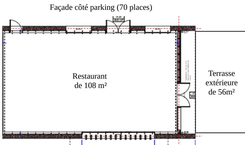
Projet Plan de masse de la cellule N°2 (restauration)
